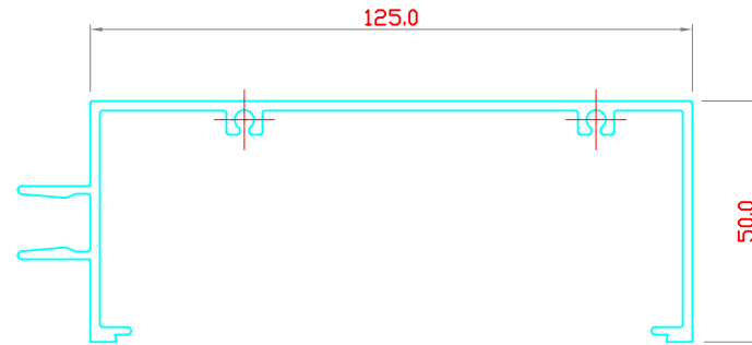
HEAD/ TRANSOM FRAME 5000-SPT01
