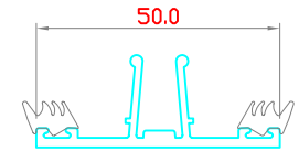
TRANSOM CAP 5000-SP16
