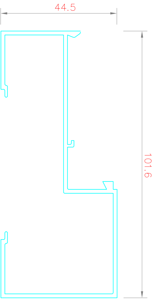
SILL / TRANSOM FRAME
